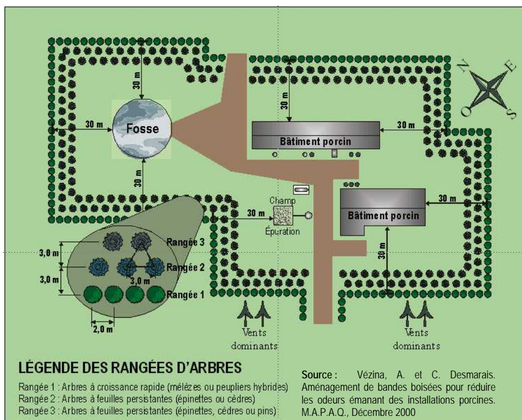
Croquis 15.1 : Schéma illustrant l'aménagement d'une haie brise-vent autour d'une installation d'élevage
